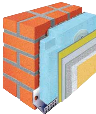
Εξιηασμένη Πολυστερίνη XPS
